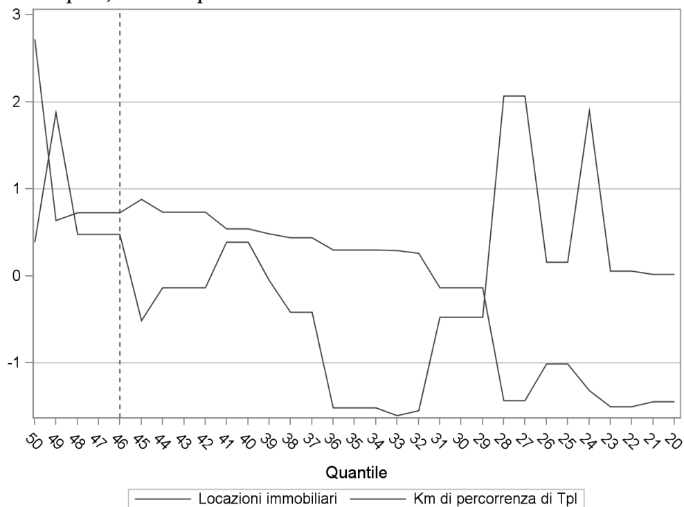
Figura A11 – Trasporti, stima dei parametri standardizzati
