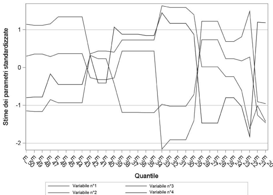
Figura A2 - Stima dei parametri standardizzati al variare del quantile q
