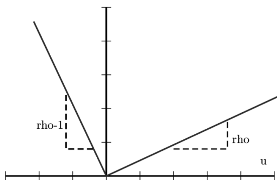
Figura A1 : Funzione \rho_q
