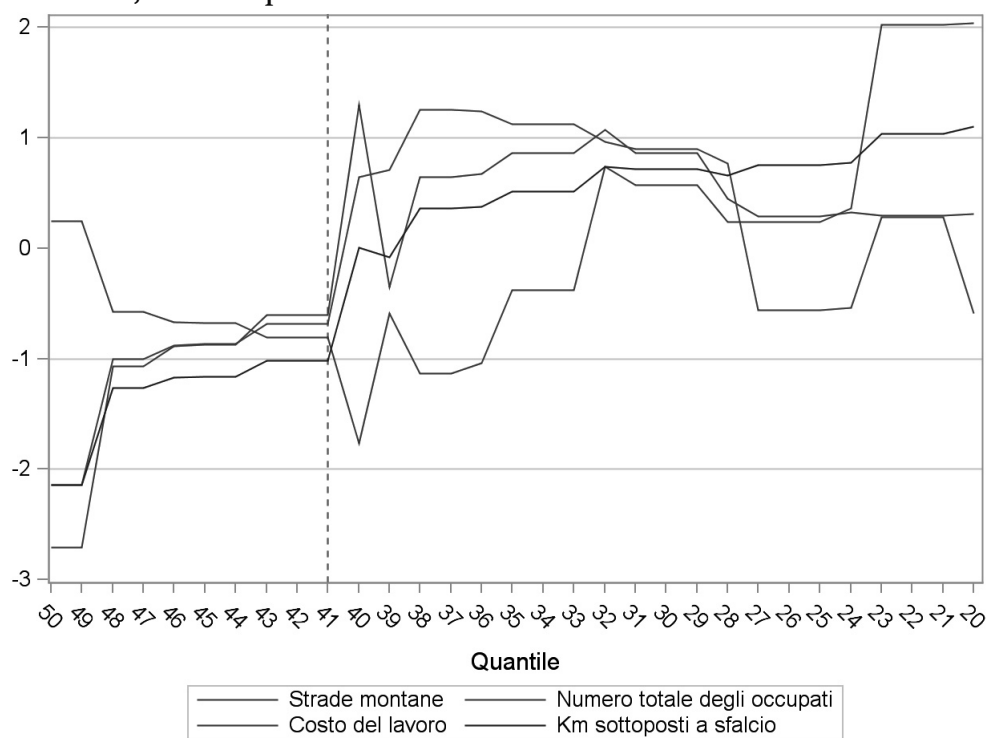
Figura A5 – Territorio, stima dei parametri standardizzati
