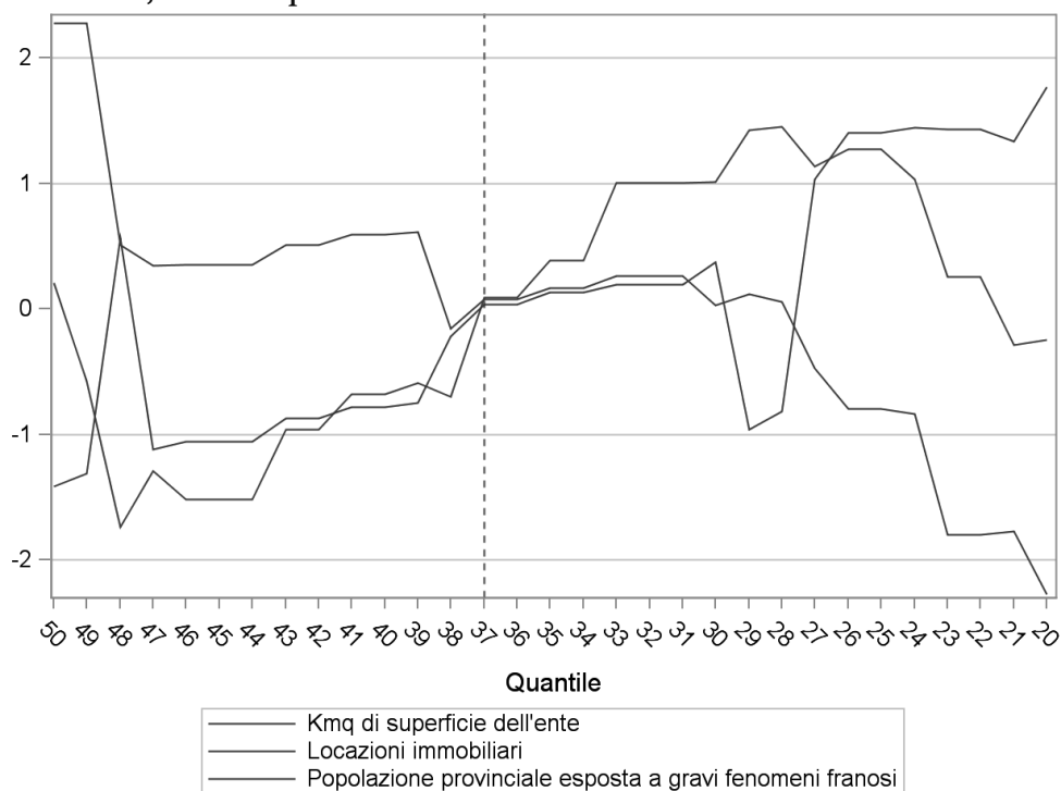
Figura A7 – Ambiente, stima dei parametri standardizzati
