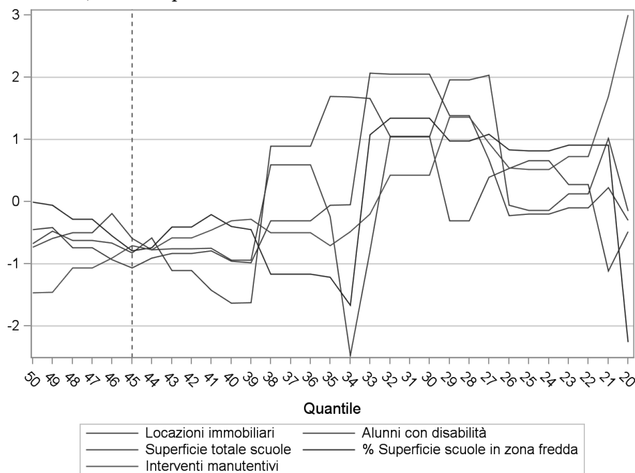
Figura A3 - Istruzione, stima dei parametri standardizzati
