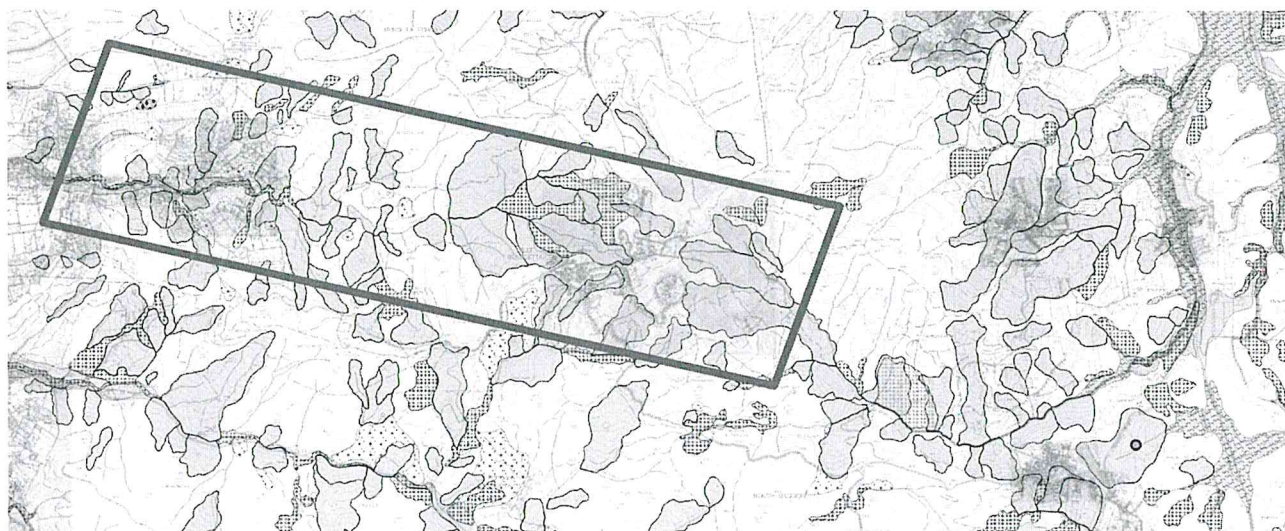
Estratto DB Geomorfologico Regione Toscana relativo alla S.P. 5 “Della Valle Benedetta” (in giallo le frane, in azzurro i depositi superficiali)
