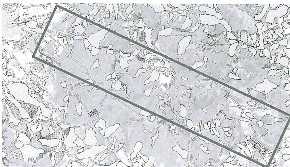
Estratto DB Geomorfologico Regione Toscana relativo alla S.P. 8 (in giallo le frane, in azzurro i depositi superficiali)
