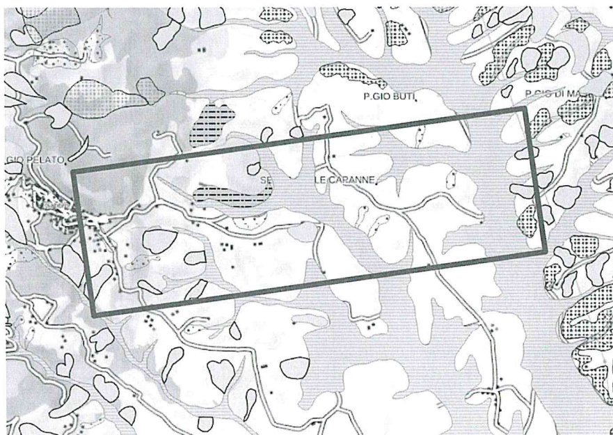
Estratto DB Geomorfologico Regione Toscana relativo alla S.P. 11 ter "Per Orciano" (in giallo le frane, in azzurro i depositi superficiali)
