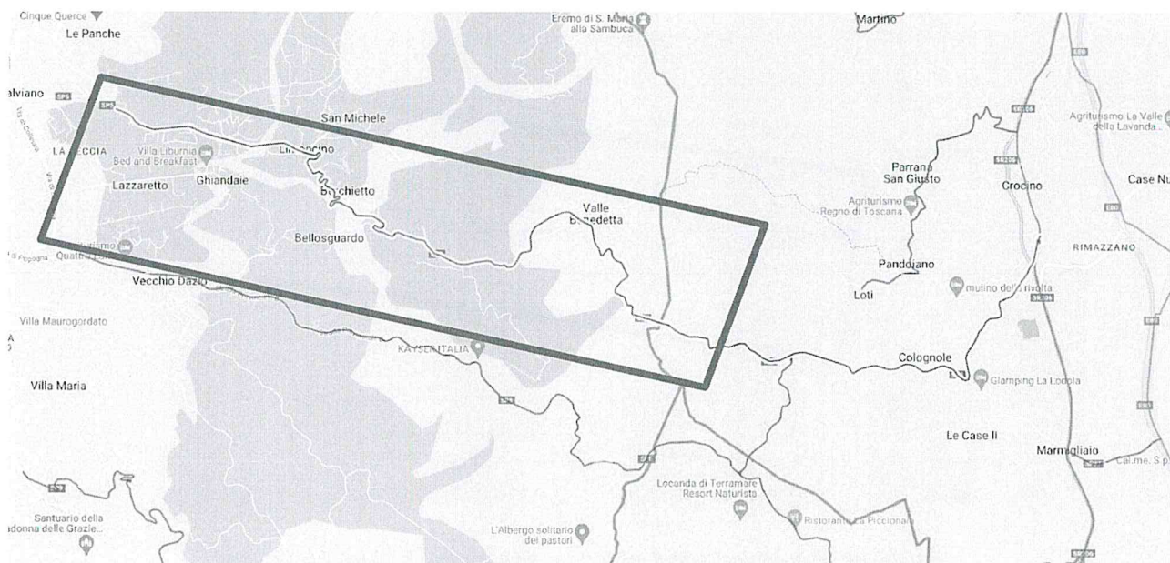
Estratto DB Geomorfologico Regione Toscana relativo alla S.P. 5 “Della Valle Benedetta” (in giallo le frane, in azzurro i depositi superficiali)
